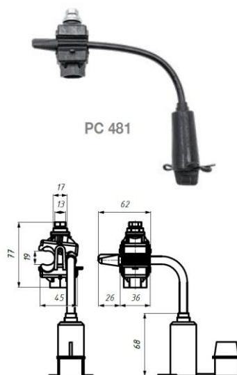
Рис. 1. Внешний вид зажима для временного заземления РС 481.
