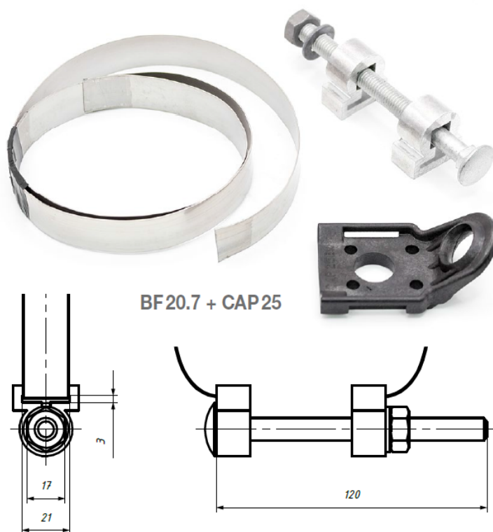
Рис. 1. Внешний вид крепежного хомута BF 20.7 + CAP 25.
