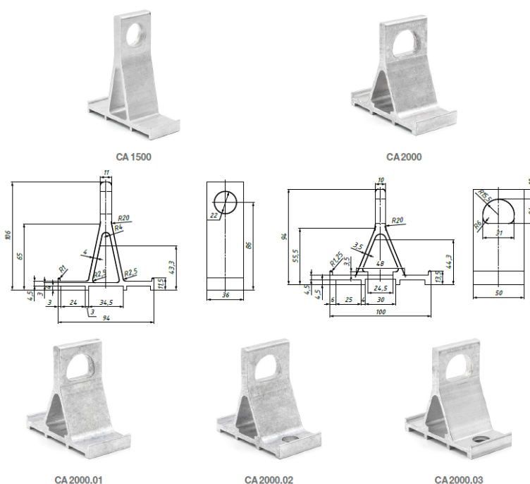
Рис. 1. Внешний вид анкерных кронштейнов СА 2000, СА 2000.01, СА 2000.02, СА 2000.03, СА 1500.
