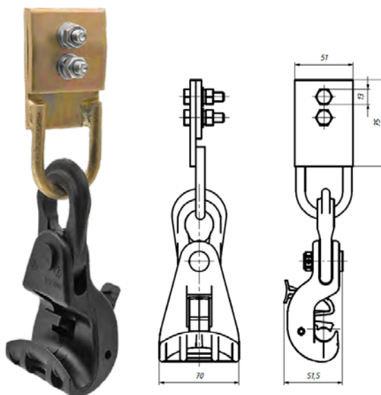
Рис. 1. Внешний вид комплекта промежуточной подвески для троса CS 2.
