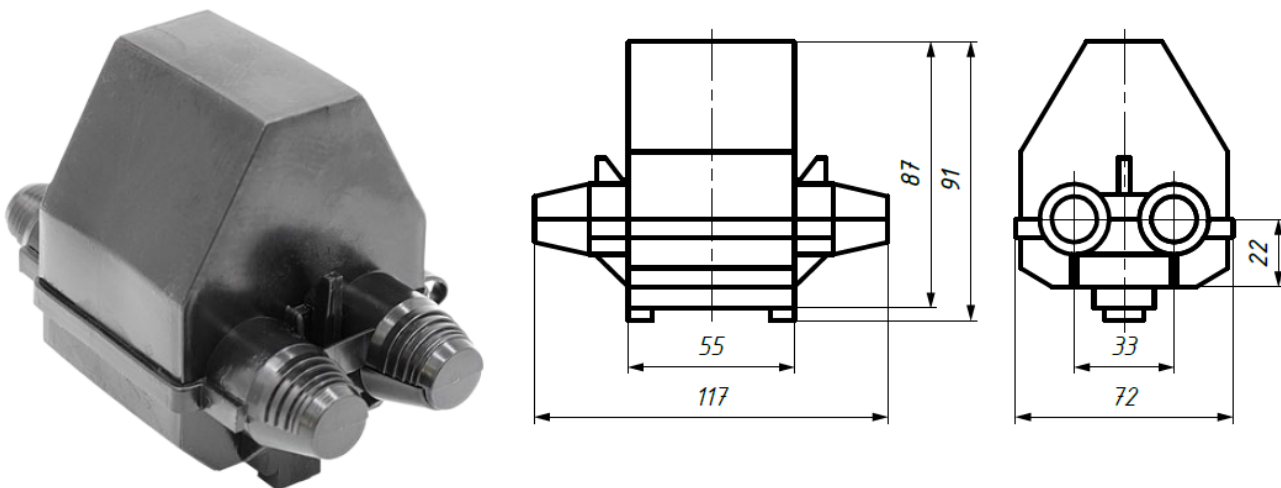
Рис. 1. Внешний вид кожуха большого К-2.
