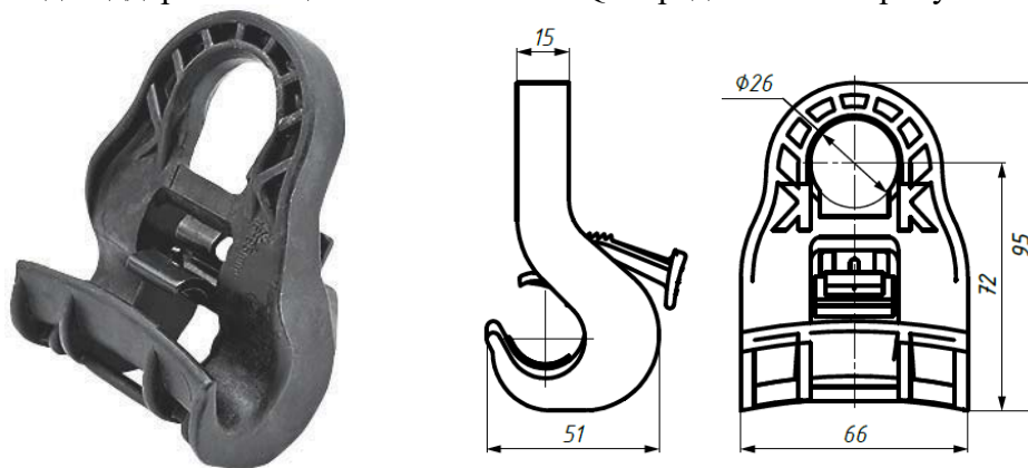
Рис. 1. Внешний вид поддерживающего зажима PS 54 QC.
