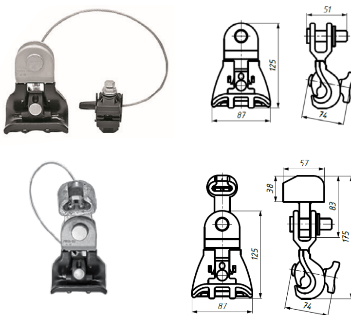
Рис. 1. Внешний вид поддерживающих зажимов PSM 25-150, PSM 25-150S.
