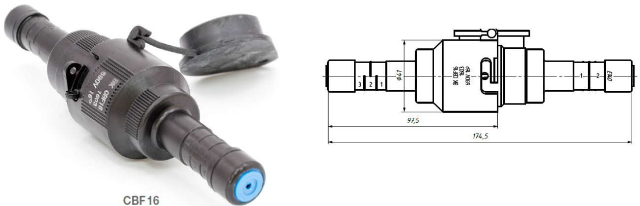
Рис. 1. Внешний вид ограничителя мощности CBF 16.
