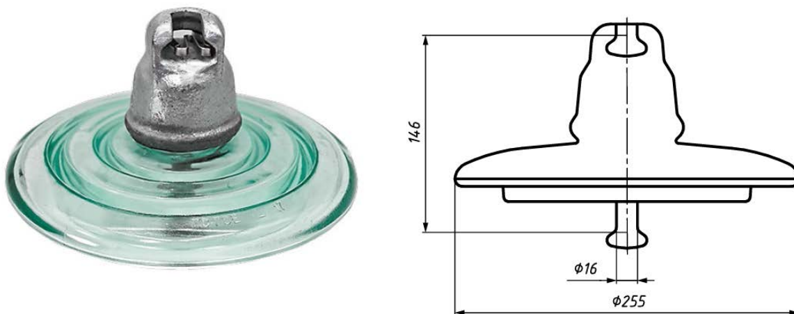
Рис. 1. Внешний вид подвесного стеклянного изолятора ПС 70Е.
