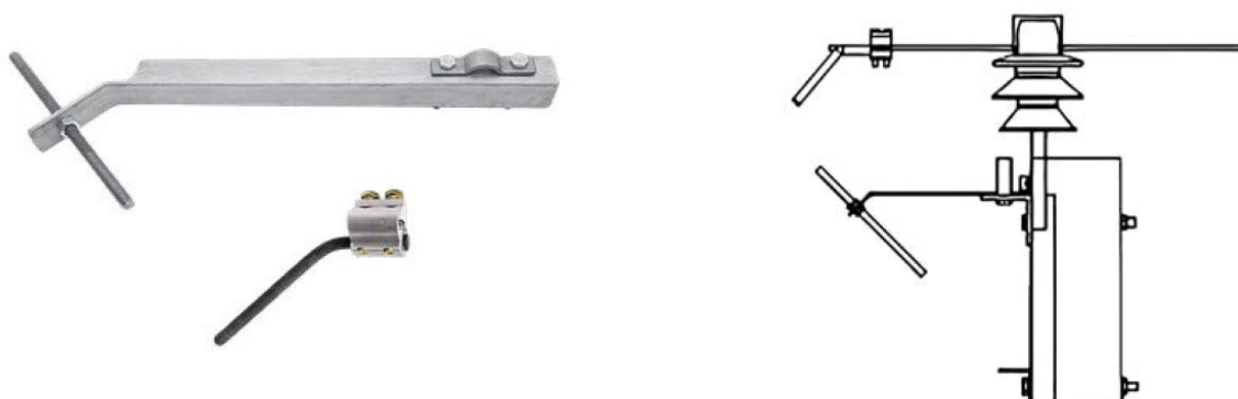
Рис. 1. Внешний вид устройств защиты от дуги APD-1.
