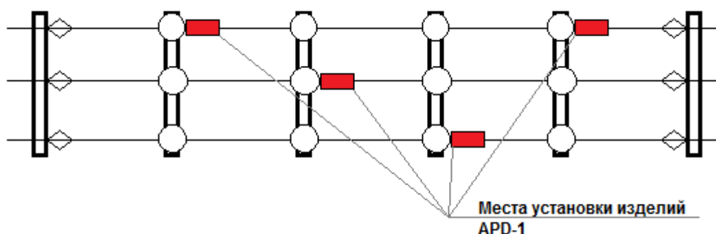
Схема 1. Схема установки устройств APD-1 на промежуточных опорах с чередованием фаз
