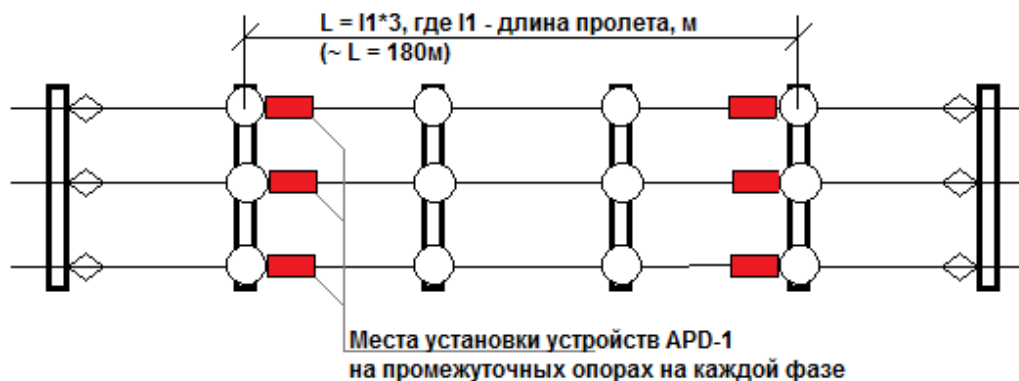
Схема 2. Схема установки устройств APD-1 на промежуточных опорах на каждой фазе
